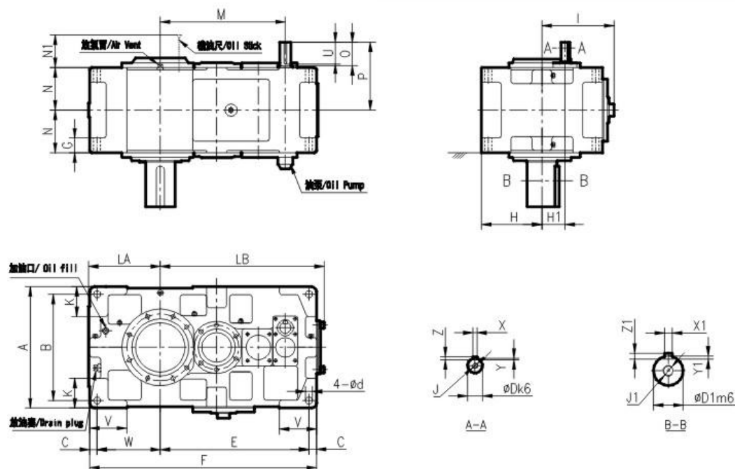
P系列TSG齒輪箱外形尺寸圖 TSG Gear Box Size Chart for Parallel Shaft
