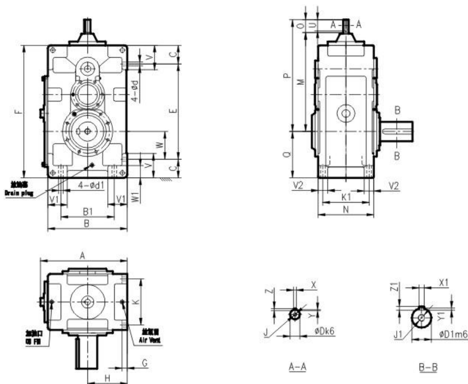
R系列TSG齒輪箱外形尺寸圖 TSG Gear Box Size Chart for Right Angle Shaft
