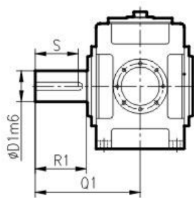
實心出力軸 Solid Output Shaft
