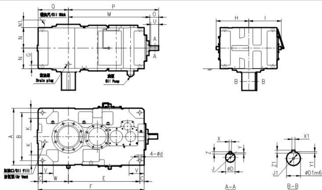
R系列TSG齒輪箱外形尺寸圖 TSG Gear Box Size Chart for Right Angle Shaft
