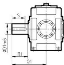
實心出力軸 Solid Output Shaft
