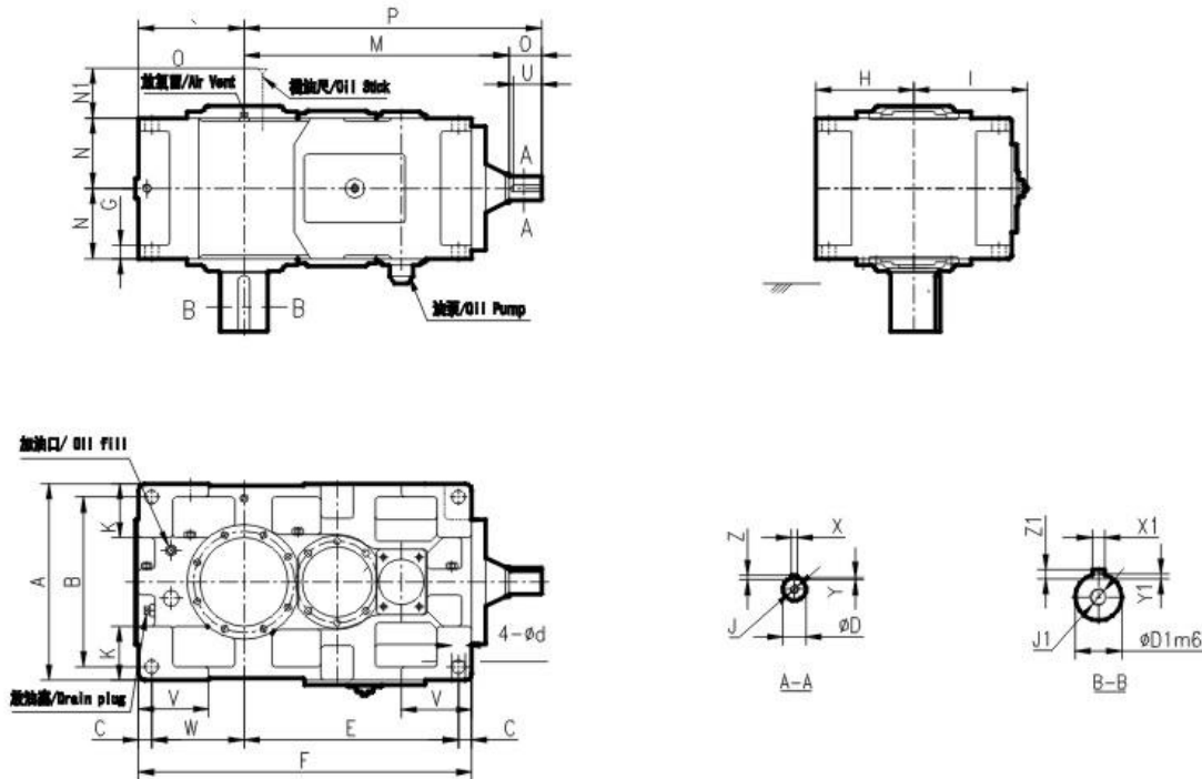
R系列TSG齒輪箱外形尺寸圖 TSG Gear Box Size Chart for Right Angle Shaft
