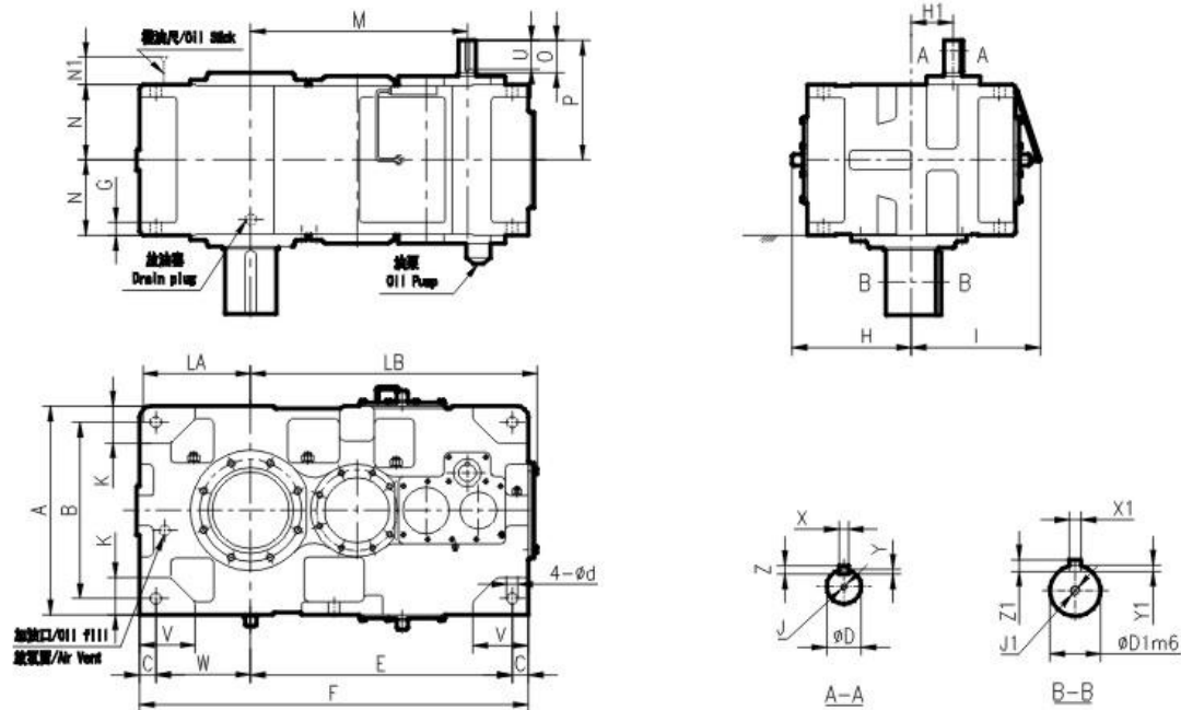
P系列TSG齒輪箱外形尺寸圖 TSG Gear Box Size Chart for Parallel Shaft
