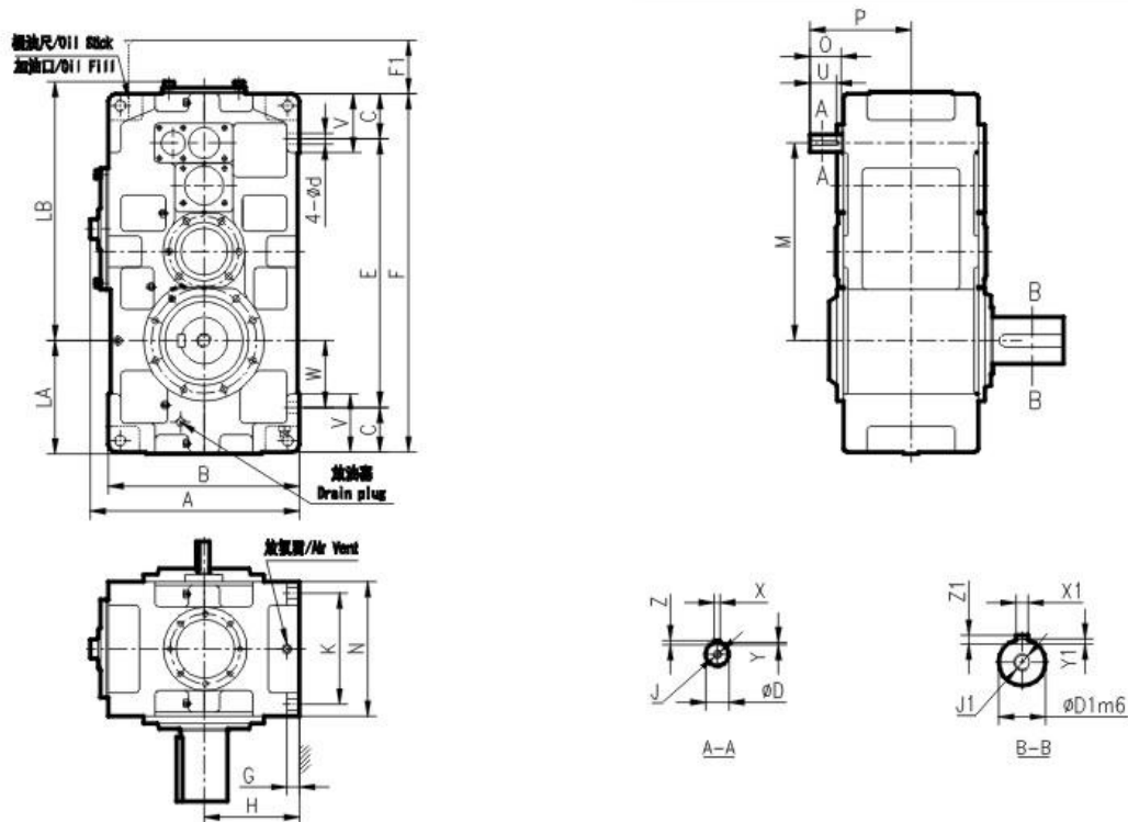
P系列TSG齒輪箱外形尺寸圖 TSG Gear Box Size Chart for Parallel Shaft
