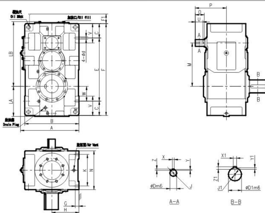
P系列TSG齒輪箱外形尺寸圖 TSG Gear Box Size Chart for Parallel Shaft
