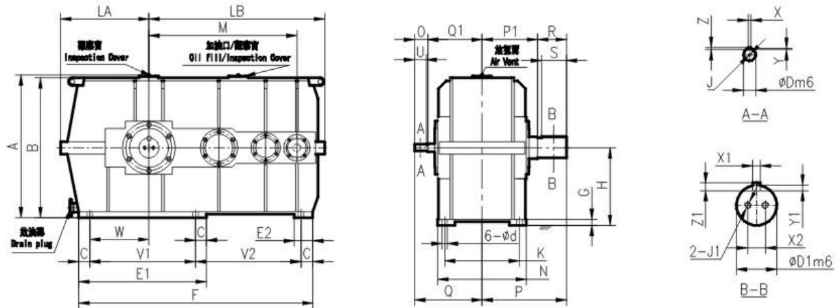
P系列TSG齒輪箱外形尺寸圖 TSG Gear Box Size Chart for Parallel Shaft
