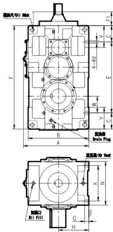
R系列TSG齒輪箱外形尺寸圖 TSG Gear Box Size Chart for Right Angle Shaft
