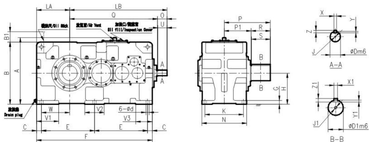
R系列TSG齒輪箱外形尺寸圖 TSG Gear Box Size Chart for Right Angle Shaft
