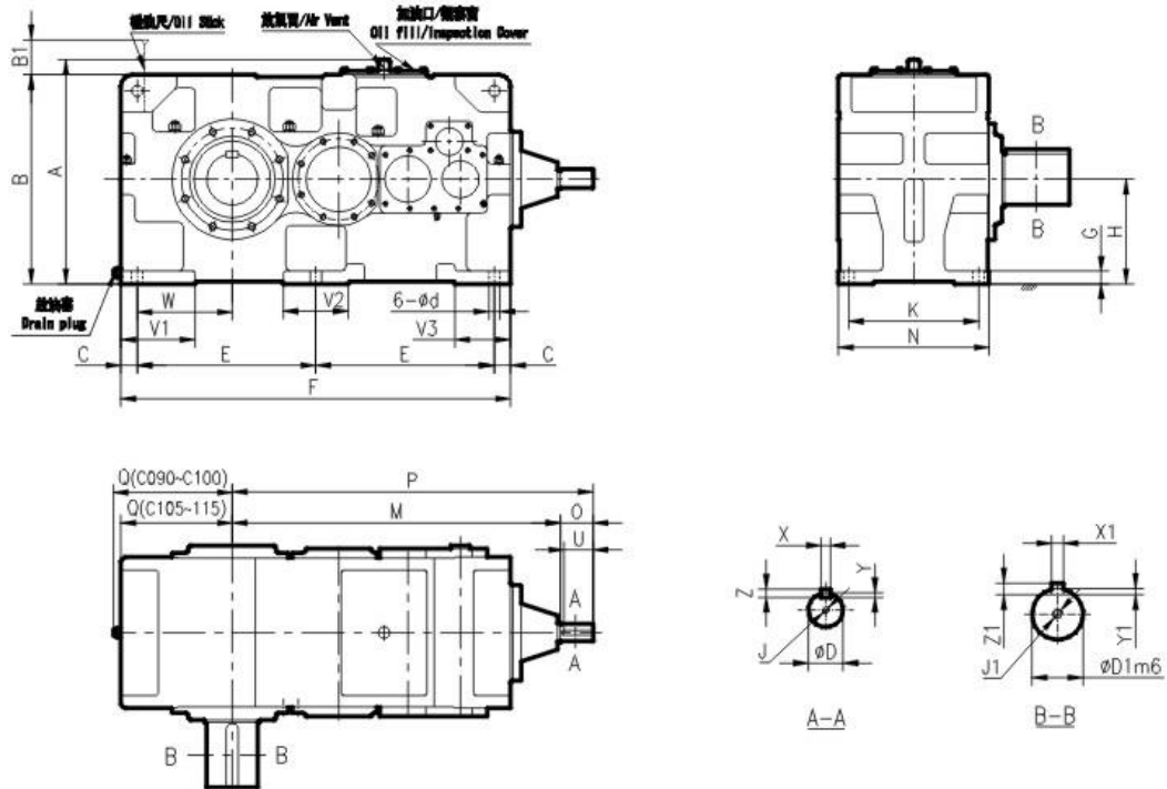
R系列TSG齒輪箱外形尺寸圖 TSG Gear Box Size Chart for Right Angle Shaft
