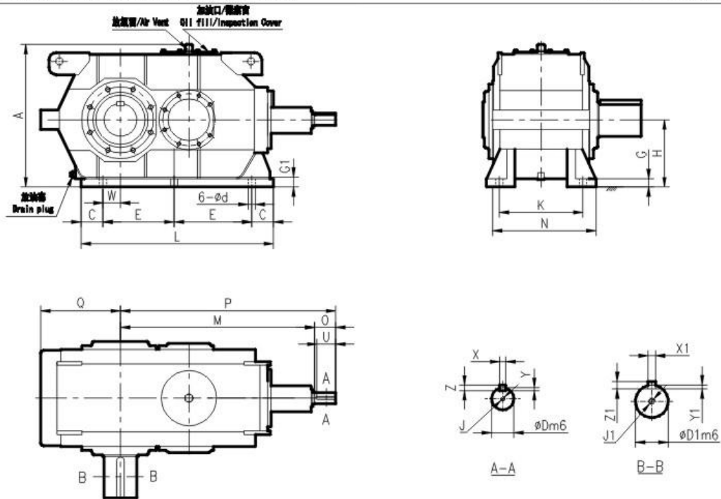
R系列TSG齒輪箱外形尺寸圖 TSG Gear Box Size Chart for Right Angle Shaft
