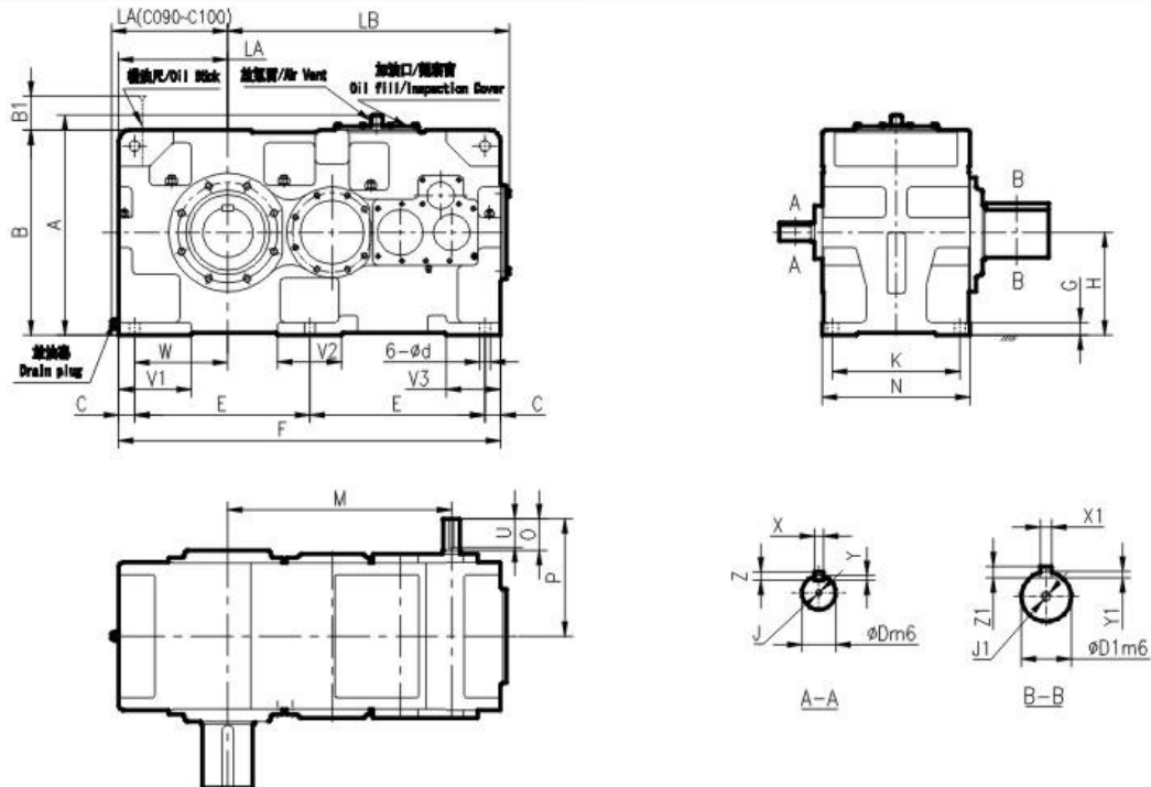
P系列TSG齒輪箱外形尺寸圖 TSG Gear Box Size Chart for Parallel Shaft
