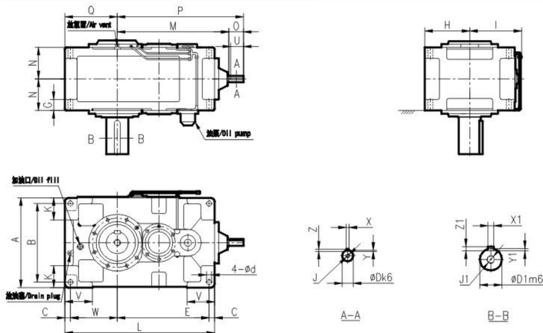
R系列TSG齒輪箱外形尺寸圖 TSG Gear Box Size Chart for Right Angle Shaft
