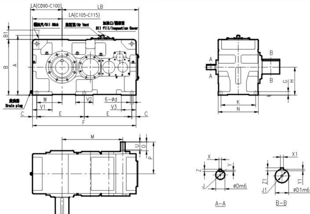
P系列TSG齒輪箱外形尺寸圖 TSG Gear Box Size Chart for Parallel Shaft
