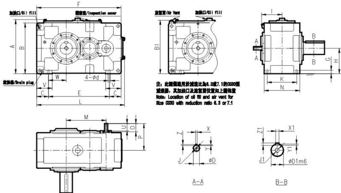
P系列TSG齒輪箱外形尺寸圖 TSG Gear Box Size Chart for Parallel Shaft
