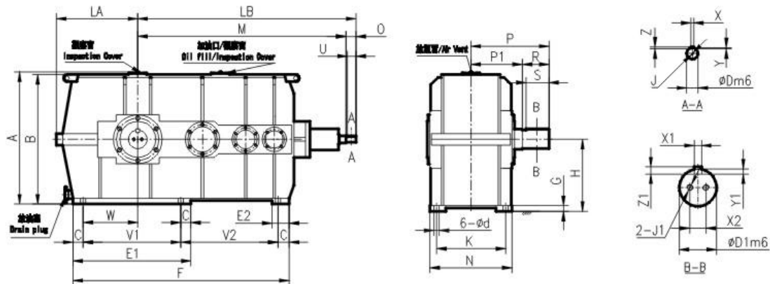
R系列TSG齒輪箱外形尺寸圖 TSG Gear Box Size Chart for Right Angle Shaft
