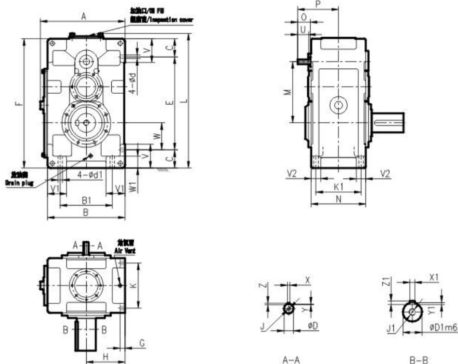
P系列TSG齒輪箱外形尺寸圖 TSG Gear Box Size Chart for Parallel Shaft
